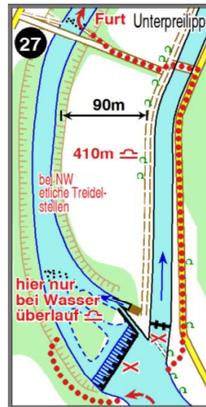
Saale km 270,5 Wehr Unterpreilipp: neue Skizze:
